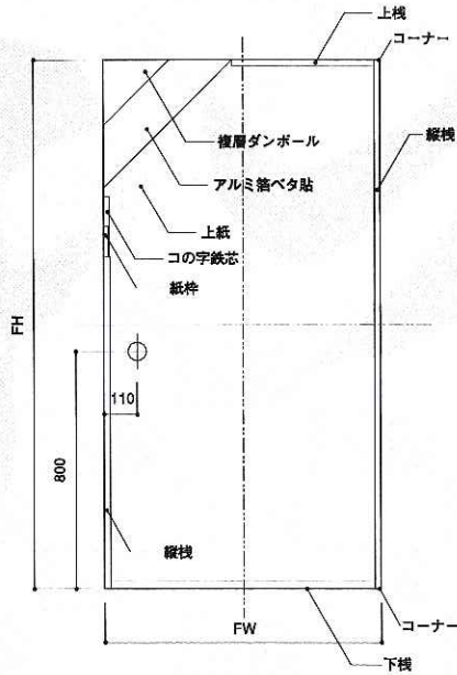
納め図
